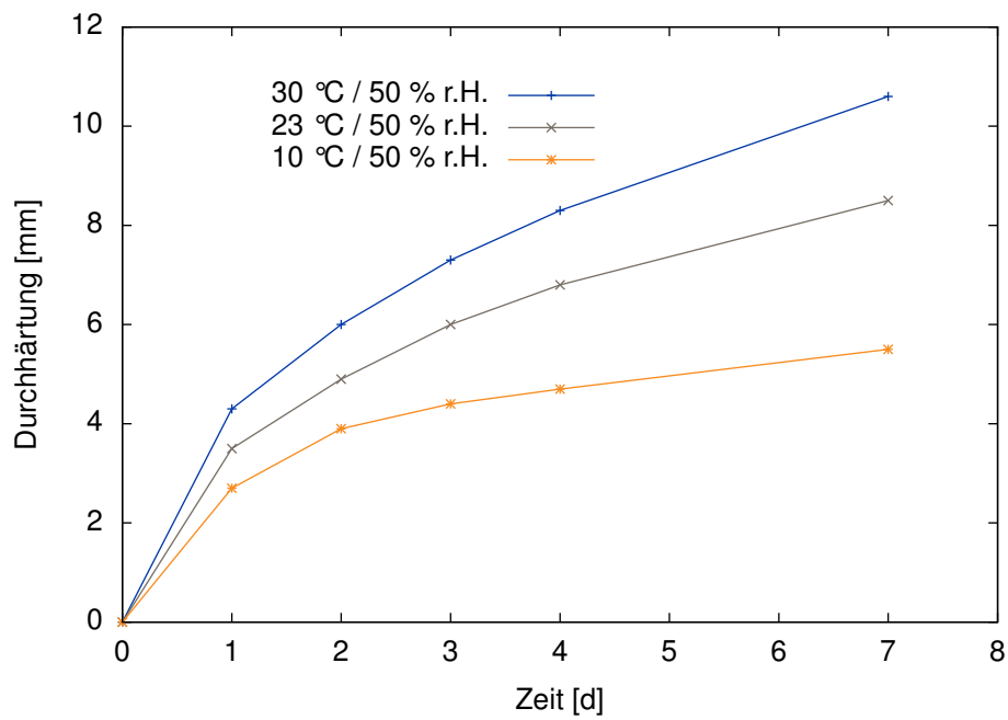
Abbildung 1: Durchhärtung des Klebstoffs in Abhängigkeit von der Temperatur
